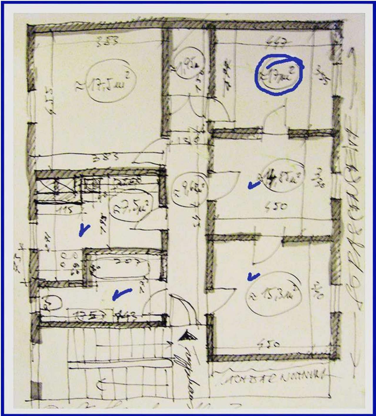
Grundriss
